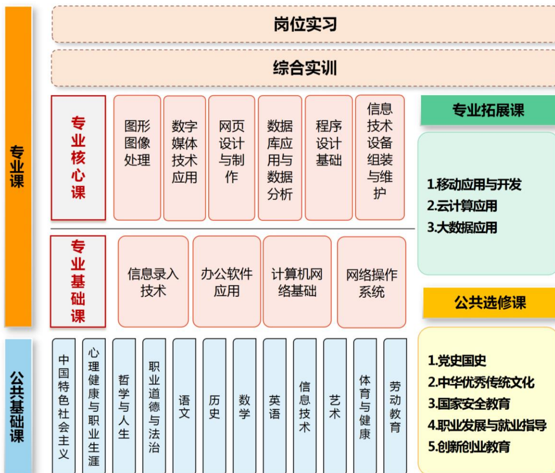
图 1 课程结构图
